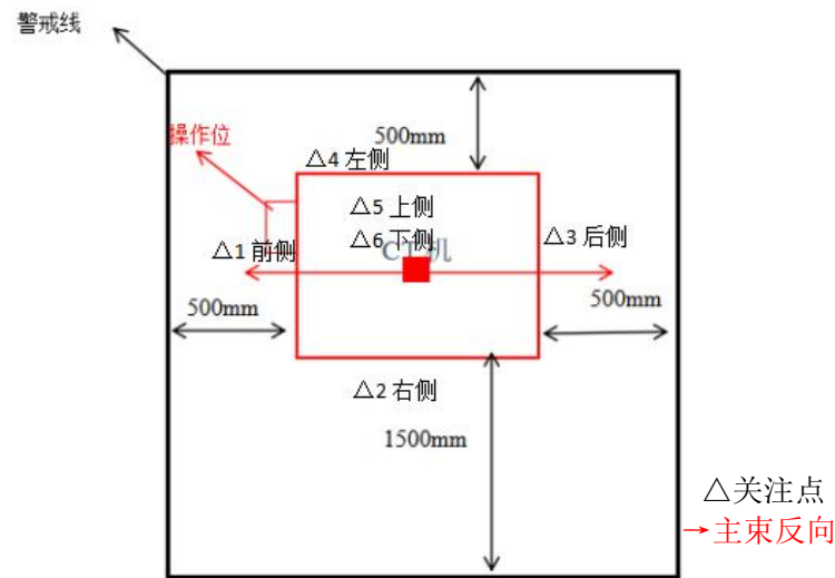
图 11-1 工业 CT 机的摆放位置图
