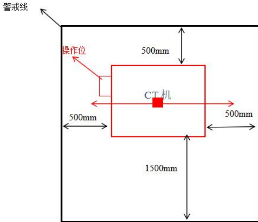
图 1-4 CT 检测区平面布置图
