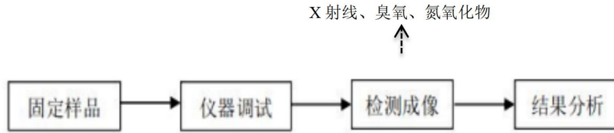
图 9-2 本项目工业 CT 机工艺流程
