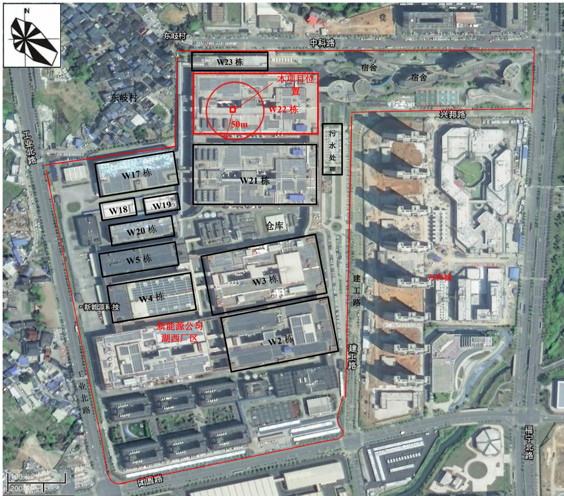
图 1-2 项目周边环境示意图及厂区平面布置图
